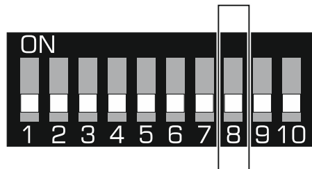
Abb. 3. Der Schalter zur Bestimmung, welche Antenne zur Übertragung benutzt werden soll.
