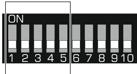
Abb. 4. DIP-Schalter zur Einstellung der Adresse, wenn das Funkbasismodul an die Zentrale INTEGRA / INTEGRA Plus angeschlossen ist.
