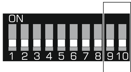
Abb. 2. Schalter zur Bestimmung des Betriebsmodus des Funkbismoduls.
