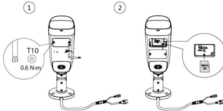
Abbildung 3-2 Einsetzen einer SD-Karte (Einheit: mm [Zoll])
