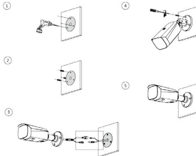
Abbildung 3.3 A - Kabeldurchführung durch die Montagefläche
