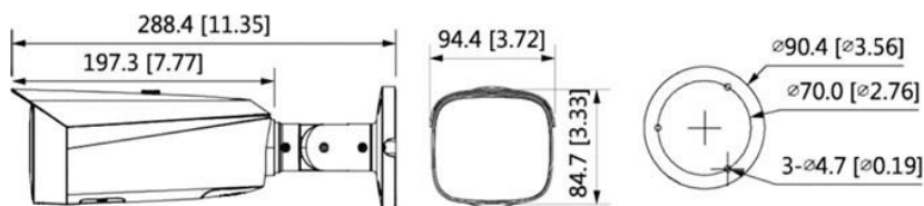
Abbildung 3-1 Abmessungen (Einheit: mm [Zoll])
