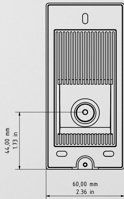
Wandmontageplatte Rückseite
