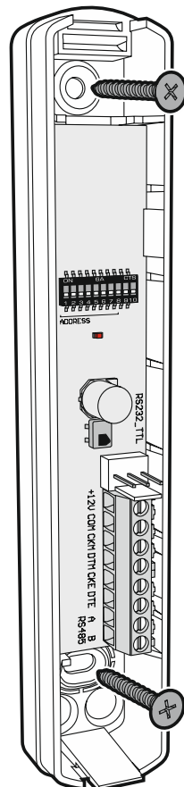
Abb. 5. Montage des Gehäuseunterteils.
