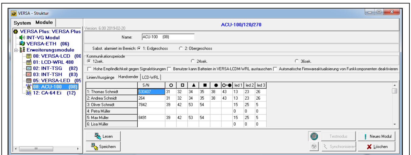
Abb. 24. Programm DLOADX: Verwaltung der Handsender beim Anschluss des Funkbasismoduls an die Zentrale VERSA / VERSA Plus / VERSA IP.
