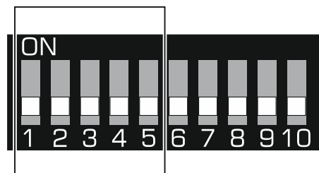
Abb. 3. DIP-Schalter zur Einstellung der Adresse, wenn das Funkbasismodul an die Zentrale INTEGRA / INTEGRA Plus angeschlossen ist.
