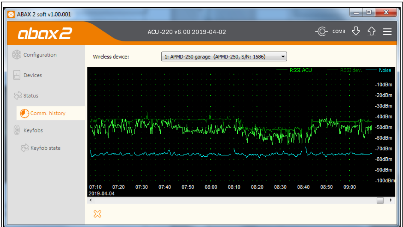
Fig. 14. ABAX 2 Soft program: “Comm. history” tab.
